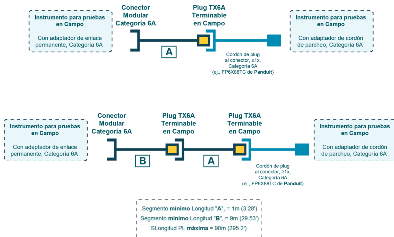
La Figura 9 muestra la representación esquemática de las pruebas a enlace permanente mediante el Modelo Alterno
